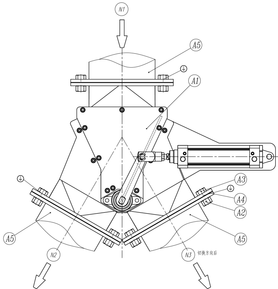
A-1 典型安装图
